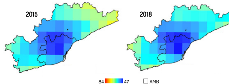
Concentració mitjana anual de O_3 ( \mu g/m^3 ) a la Regió Metropolitana de Barcelona (RMB) 2015 i 2018
