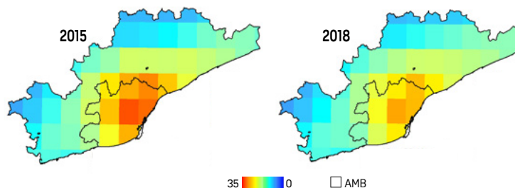
Concentració mitjana anual de PM_{2,5} ( \mu g/m^3 ) a la Regió Metropolitana de Barcelona (RMB) 2015 i 2018
