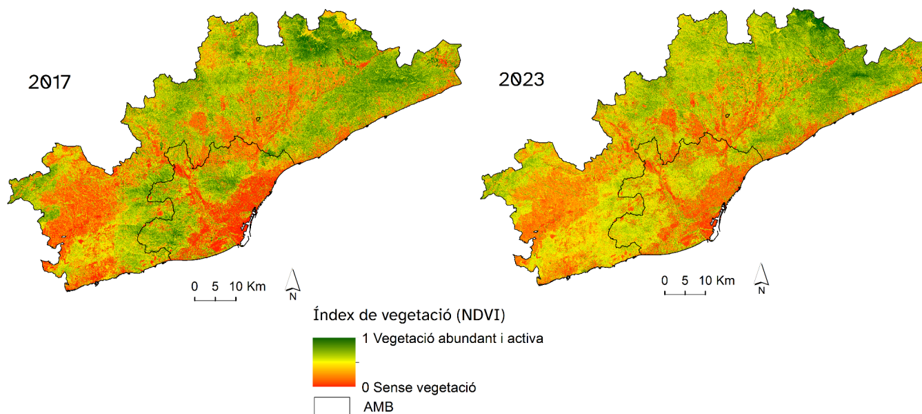
Valor mitjà anual de l'índex de vegetació NDVI a la Regió Metropolitana de Barcelona (RMB), 2017 i 2023
