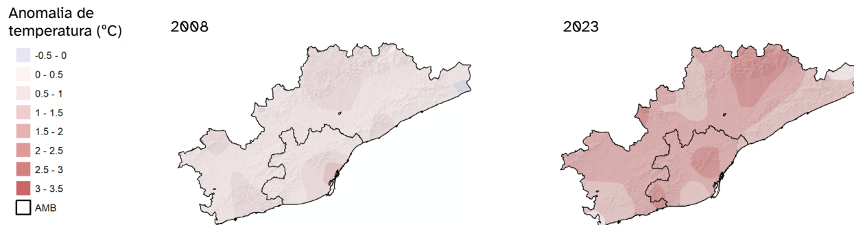
Anomalia de temperatura i de precipitació a La Regió Metropolitana de Barcelona (RMB), 2008 i 2023
