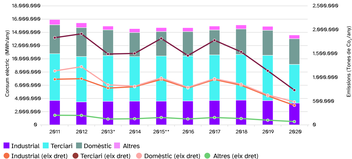
Consum elèctric per sector i emissions de CO 2 associades a l'àmbit de l'AMB, 2011-2020
