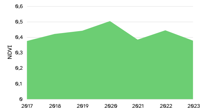
Valor mitjà anual NDVI a la RMB, 2017-2023
