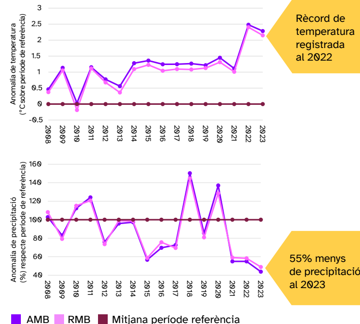
Evolució de l'anomalia de temperatura i de l'anomalia de precipitació a la RMB i l'AMB entre, 2008-2023
