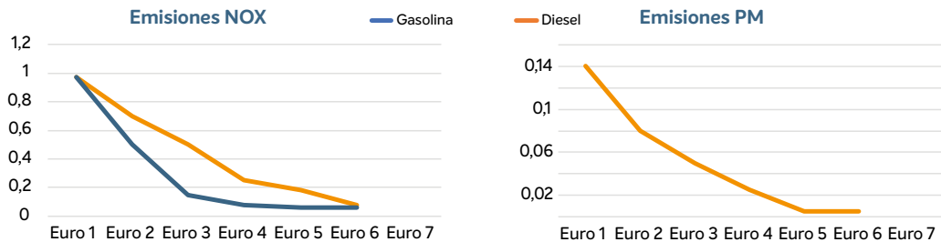
Figura 23. Emisiones NOx y Emisiones PM (g/km)
